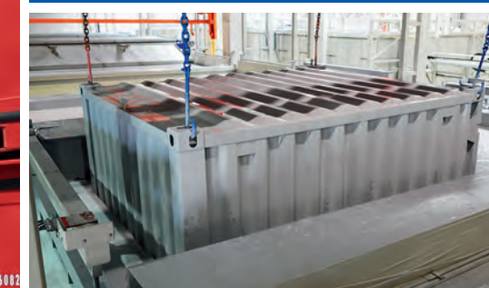
KTL-základní nátěr v ponorné vaně
