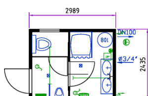
Sanitärcontainer 10'
