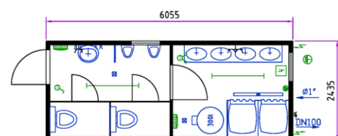
Sanitärcontainer 20'
