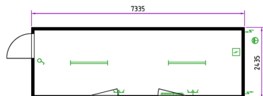
Bürocontainer 24'
