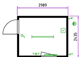
Bürocontainer 20'
