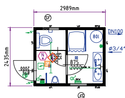
Bungalow sanitaire 10'
