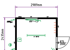
Bungalow bureau 10'
