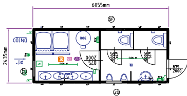
Bungalow sanitaire 20'
