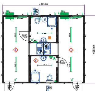
Unité de logement 3x20'
