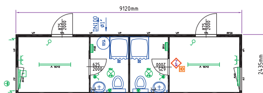
Unité de logement 1 x 30'
