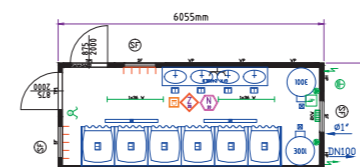
Tuš-kontejner 20'
