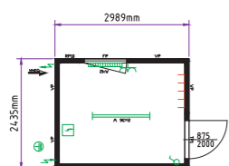
Uredski kontejner 10'
