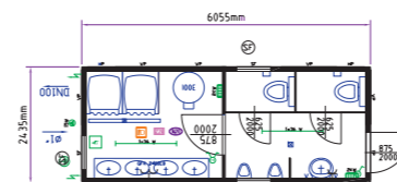
Sanitarni kontejner 20'
