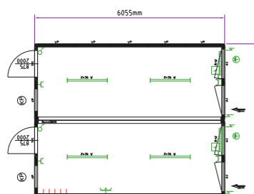
Dupla egység 20' irodakonténer
