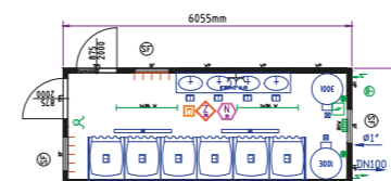
20' zuhanyzó konténer
