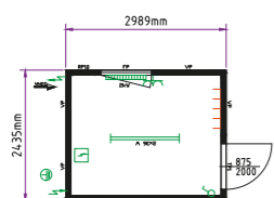
10' irodakonténer
