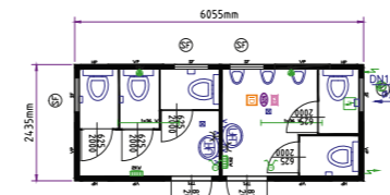
20' női/férfi WC konténer
