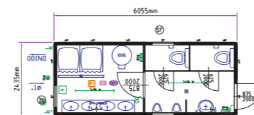
20' szaniterkonténer
