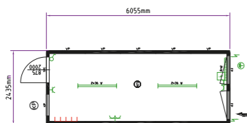
20' irodakonténer
