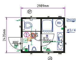
10' szaniterkonténer
