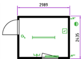
Kantoorunit 10'
