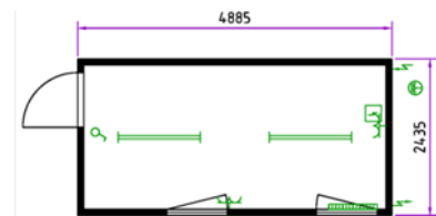
Kantoorunit 16'
