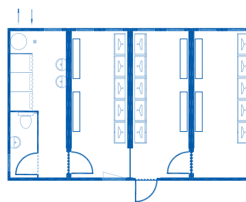
Szatnie z pomieszczeniem sanitarnym dla klubów sportowych
