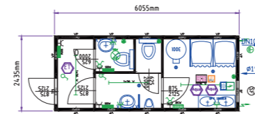
Kontener sanitarny 20'
