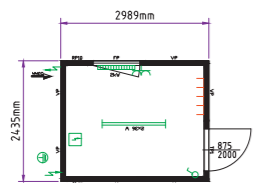
Kontener biurowy 10'
