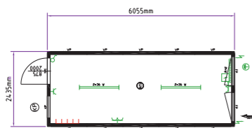
Kontener biurowy 20'
