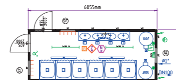
Kontener prysznicowy 20'
