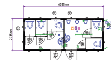
WC kontejner ženski/moški 20'
