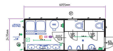
Sanitarni kontejner 20'
