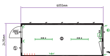
Kontejner pisarna 20'
