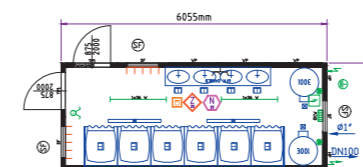
Kontejner 20' za prhanje
