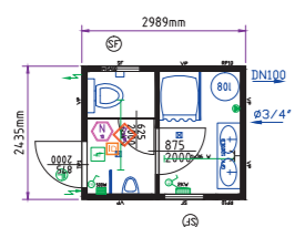
Sanitarni kontejner 10'
