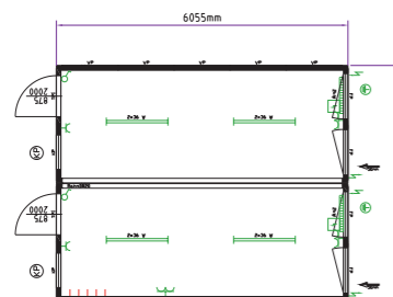
Pisarniški kontejner dvojni sklop
