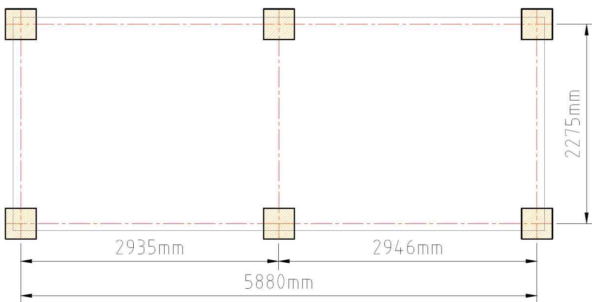
Abbildung 6: 20' Fäkalientank
