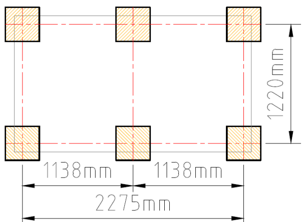
Abbildung 4: 8' Fäkalientank mit 1x oder 2x BM/SA-Box 5'
