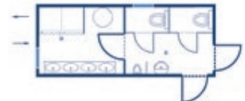
20' vegyes szaniterkonténer
