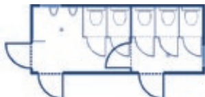
20' vegyes WC-konténer
