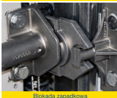
Blokada zapadkowa
