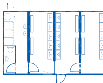
Garderobe s sanitarnim prostorom za športna društva
